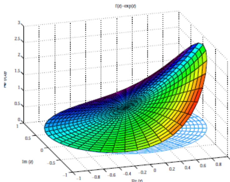
Gráfica de la función parte real de \exp(z) , z \in D(0; 1) := \{z \in \mathbb{C}; |z| \leq 1\}
